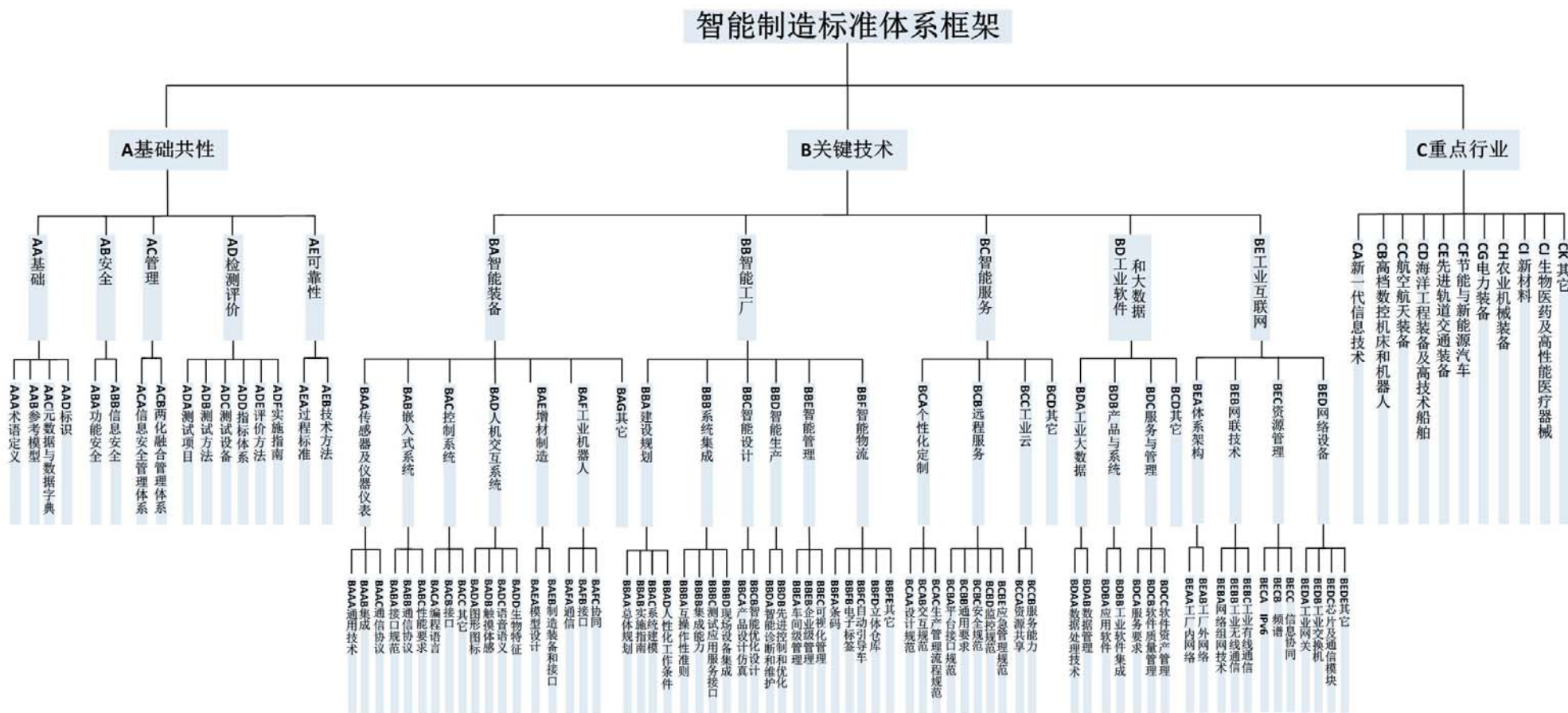
图 6 智能制造标准体系框架
